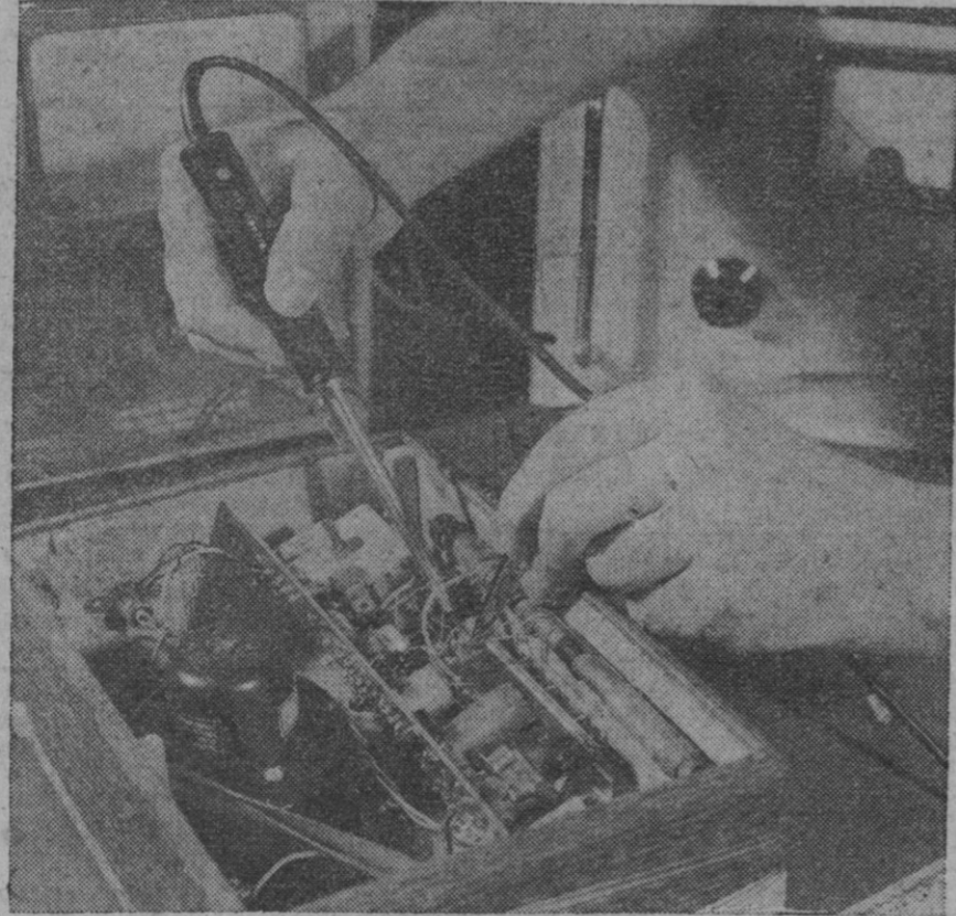
Este nuevo soldador, que opera con una potencia de quince vatios tomada de la línea principal, ha sido introducido al mercado por una compañía británica de electricidad. No mide más que 215,9 mm. de longitud, y su peso es de poco más de ochenta y cinco gramos. El remate de cobre cromado tiene un diámetro de solo 3,75 mm., lo que hace a este hierro particularmente apto para operar en espacios cerrados, así como para soldar accesorios de tipo miniatura, que pudieran correr riesgo de ser dañados por la aplicación de calor excesivo
