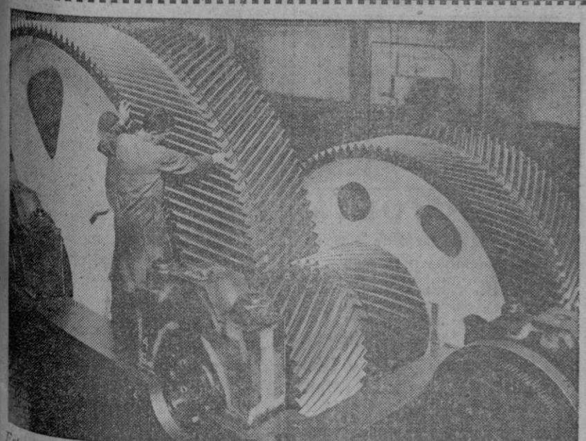
Estos engranajes de doble reducción, pesan doscientas toneladas. Están siendo sometidos a la inspección final, antes de ser desmontados y remitidos a una acería para usarse en un nuevo tren laminador. Se emplearon dos grúas de treinta y cinco toneladas, en tándem, para manejar los engranajes mayores, y la película de aceite de alta presión, bombeada a conchas especiales de cojinetes, para soportar el peso de las ruedas mientras que se equilibraban con mucha precisión, permitió mover los engranajes meramente con la punta de los dedos
