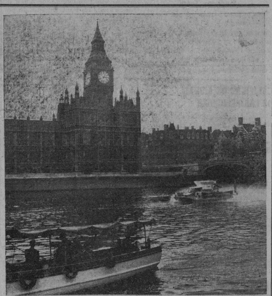
El S. R. N. 1 "Hovercraft" británico, pilotado por el capitán de corbeta Peter Lamb, jefe de pilotos de prueba de los constructores—Saunders-Roe—forma una nube de espuma, viniendo así a interrumpir el tranquilo fluir de las aguas del Támesis frente al Parlamento, en una reciente demostración. El S. R. N. 1 tiene ahora dos motores: el originario, de pistones, para formar el "almohadón" de aire, y uno auxiliar de reacción, que provee adicional fuerza propulsora
