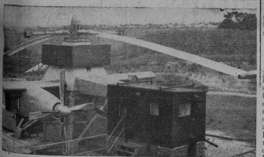
Se espera que este verano realizará su vuelo inaugural el helicóptero británico Fairey "Rotodyne", que es el mayor del mundo. Está ya a punto de terminarse la construcción de los helicópteros "Rotodyne" y actualmente se llevan a cabo pruebas en una instalación giratoria. Esta fotografía recoge un momento de las pruebas del motor de estribor y de dos palcas del rotor. El "Rotodyne" es de diseño revolucionario y combina las ventajas de las aviones de ala fija con las de aparatos de ala giratoria. Transportará a cuarenta y ocho pasajeros a velocidades de hasta 272 kilómetros por hora en trayectos de 640 kilómetros.
