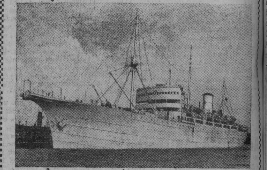
El buque destaca su silueta elegante y la valentía de su aguda pro. Pero no se trata, como pudiera parecer a primera vista, de un yate de recreo, sino de un buque cableero que, según indica su nombre, está diseñado, construido y equipado para proveer al tendido y reparación de los cables submarinos.
