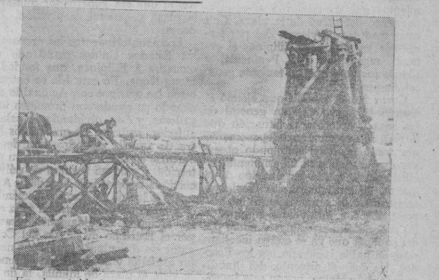
En el restablecimiento de las comunicaciones en Rusia, a muchos grados bajo cero, trabajan los pontoneros alemanes. La foto nos muestra la reconstrucción de un puente en un importante centro de carreteras
