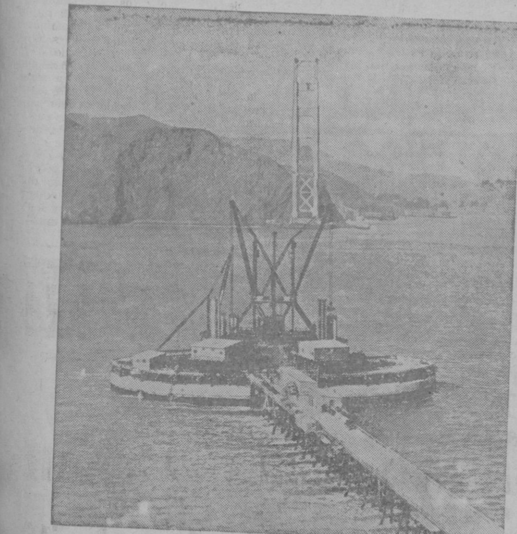
EL MAYOR FUENTE FLOTANTE DEL MUNDO. —A la entrada del puerto de San Francisco, se está construyendo el más alto puente flotante del mundo, que será denominado «La Puerta Dorada». Un aspecto de la construcción. Al fondo una de sus gigantescas torres.
