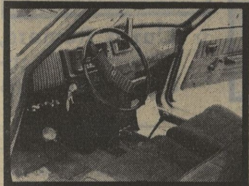
En la prueba de frenos se ha utilizado un decelerógrafo y un palpador acoplado al pedal del freno.
