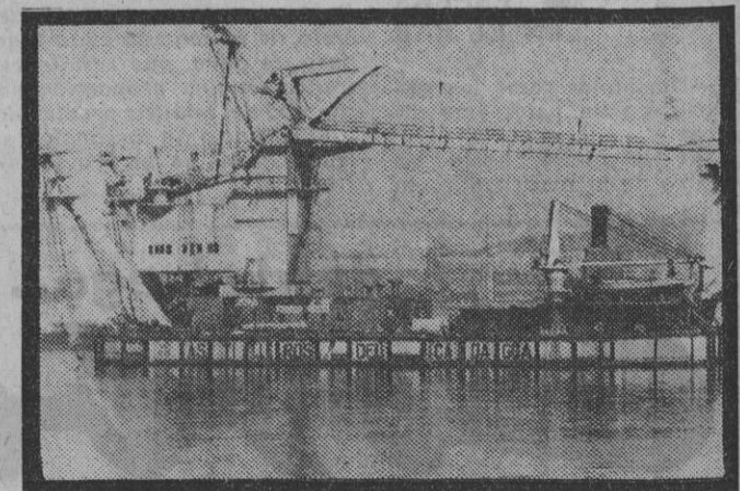
GALDAMES (Vizcaya).— Grúa gigante construida para el Iraq por las empresas Babcock & Wilcox y Astilleros Cadagua. Pesa tres mil toneladas, su capacidad de elevación es de 350 toneladas hasta una altura de 56 metros sobre el nivel del mar y va montada en una plataforma de 1.800 metros cuadrados, con cuatro metros de calado. Su importe se eleva a 250 millones de pesetas. (Telefoto Cifra Gráfica.)
