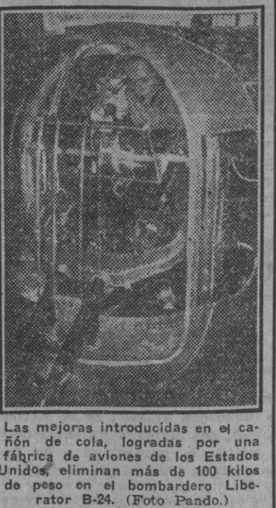
Las mejoras introducidas en el cañón de cola, lograda por una fábrica de aviones de los Estados Unidos, eliminan más de 100 kilos de peso en el bombardero Liberator B-24. (Foto Pando).
