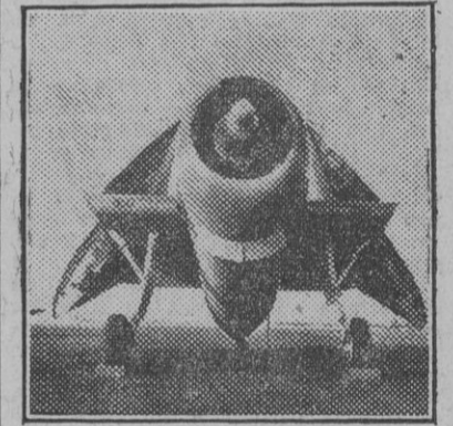
Las alas de este avión torpedero pueden plegarse en pocos segundos. En el depósito se aloja el torpedero, que ha de lanzarse a escasa altura. (Foto Pando.)
