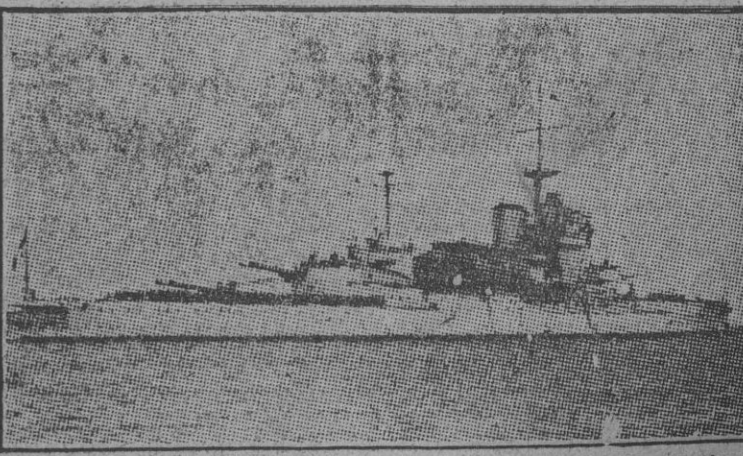
Buque de guerra del tipo "Warspite", cuyo nombre no se ha precisado aún, hundido por los japoneses en la batalla del mar del Coral. Tenía un desplazamiento de 30.800 toneladas y contaba con 1.000 hombres de dotación. Su armamento estaba compuesto de ocho cañones de 381 milímetros, 12 de 114, cuatro de 47, 32 anti-aéreos de 40 y una catapultas. Al mismo tipo pertenecía también el "Queen Elizabeth".
