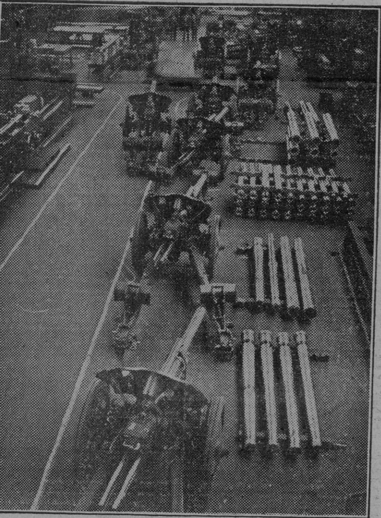
Obuses ligeros de campaña terminados en la galería de montaje.
