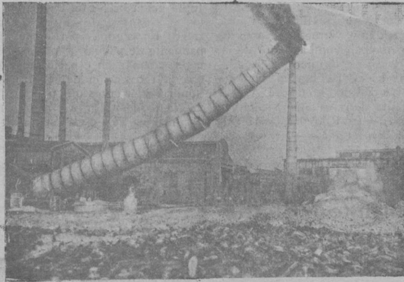
Esta gran chimenea estaba emplazada en Spandau (Berlín) y hubo necesidad de derribarla. Los obreros extrajeron ladrillos de su base y los sustituyeron por bloques de madera impregnados de petróleo. Después prendieron fuego a éstos, y la enorme chimenea vino a tierra.
