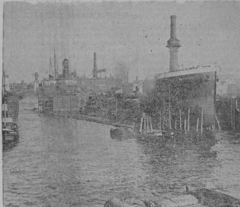
UN BARCO EN TRES TROZOS.—El vapor «Svithiod» de la Sdad. alemano-americana de petróleos, ha sufrido en los astilleros de Hamburgo una curiosa operación. La substitución de su parte central. Por lo visto la parte anterior y posterior del buque se encontraban en perfecto estado, mientras la parte central o sea la que contenía los tanques estaban sumamente averiada. La Cía. no ha creído el problema insoluble. Ha cambiado la parte central cortando el barco como si se tratase de una longaniza. Momento de ser colocada la nueva parte central.
