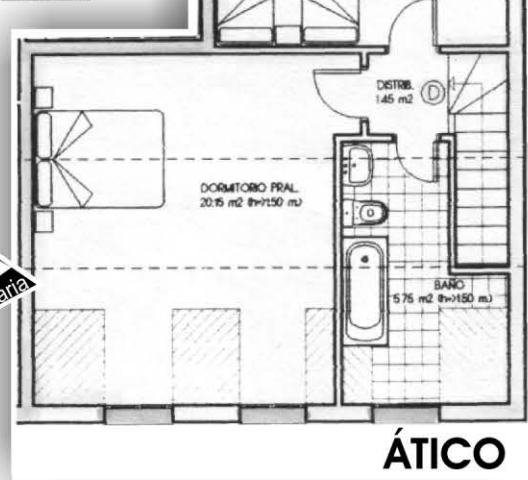
PLANTA ALTA
