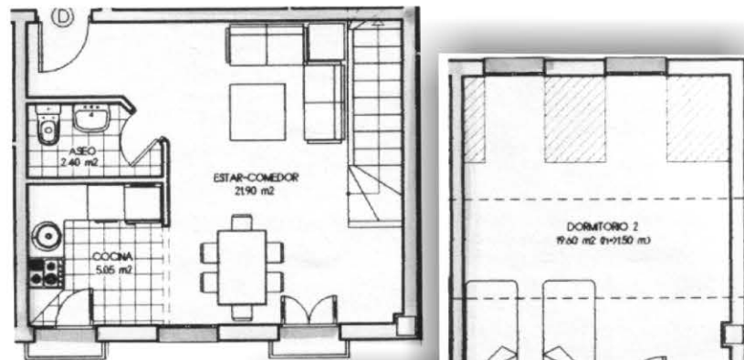
PLANTA ALTA
