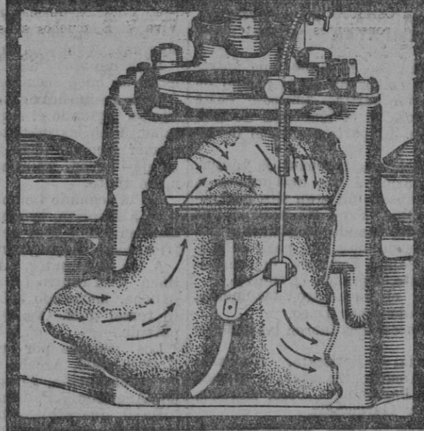
El regulador del calor de la mezcla facilita el rápido calentamiento del motor, asegurando mejor rendimiento en verano y en invierno.
