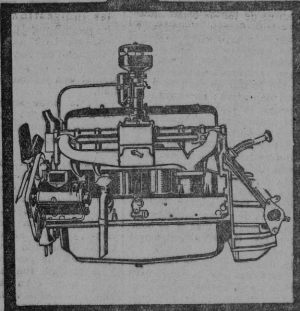
El motor de seis cilindros desarrolla ahora 53 H. P. a 2.800 revoluciones por minuto sin aumento de su fuerza fiscal (20 H. P.).
