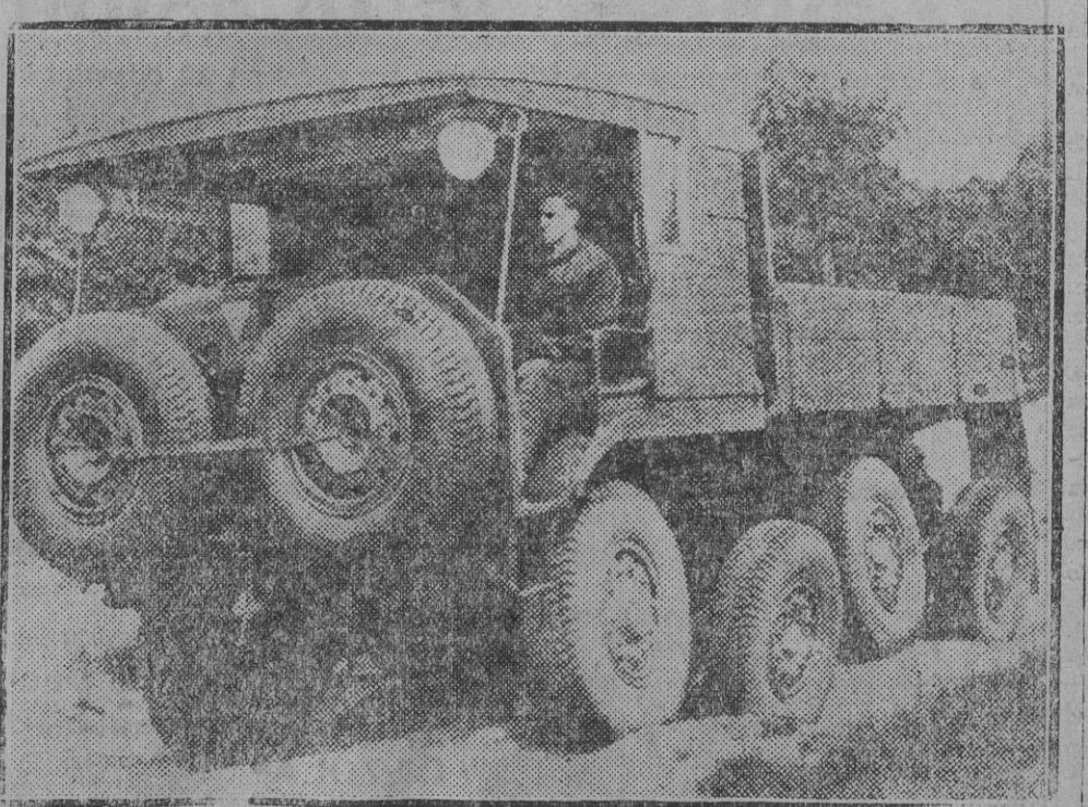
Progresos en la construcción de los automóviles.—Un autocamión cuya independencia de ruedas le permite adaptarse a las mayores desigualdades del camino.
