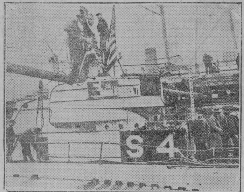
El submarino norteamericano «S-4» hundido en diciembre último que ha sido sacado a flote después de laboriosos esfuerzos. La catástrofe costó la vida de 42 hombres, ocho de cuyos cadáveres encierra todavía el sumergible.
