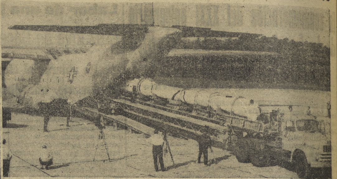
Un vehículo de lanzamiento tipo Scout es montado en un avión de transporte C-130, de las Fuerzas Aéreas de los Estados Unidos, para su traslado desde Wallops Island hasta Hampton, en Virginia. Es esta la primera vez que un Scout completamente ensamblado es transportado por aire. Se busca con ello desarrollar la técnica del transporte para las operaciones de lanzamiento de la Administración Nacional de Teronáutica y del Espacio. El cohete, que mide 21,6 metros, pesa junto con su transporte, alrededor de 31.500 kilos.
