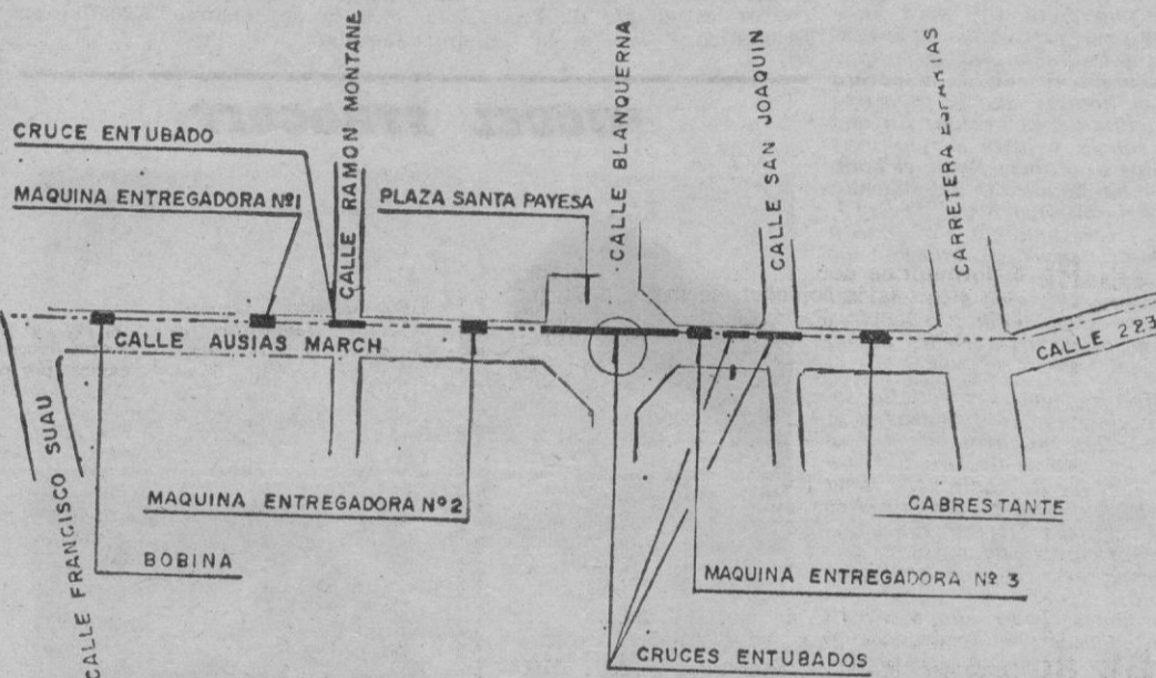
PLANO DEL LUGAR EN DONDE ESTA MISMA MAÑANA SE PROCEDERA A LA INSTALACION MECANICA DE UN TENDIDO DE CABLES SUBTERRANEOS A 66.000 VOLTIOS ANTE MAS DE 100 TECNICOS DESPLAZADOS A PALMA ESPECIALMENTE.
