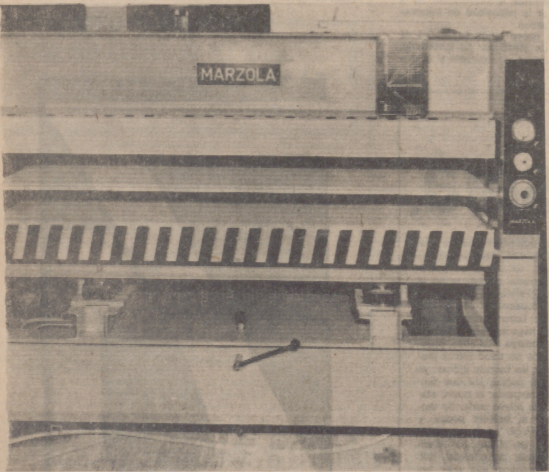
En la reciente Feria del Mueble de Valencia, Marrodán y Rezola, S. A., de Logroño, ha presentado su nueva gama de prensas hidráulicas automáticas para la industria de la madera. Cabe destacar el éxito de su modelo S-E, con calefacción por platos eléctricos Elikton, que por lo reducido de su consumo, sin instalación complementaria de caldeo, es sin duda la Prensa Ideal para la pequeña y mediana empresa de este ramo.
