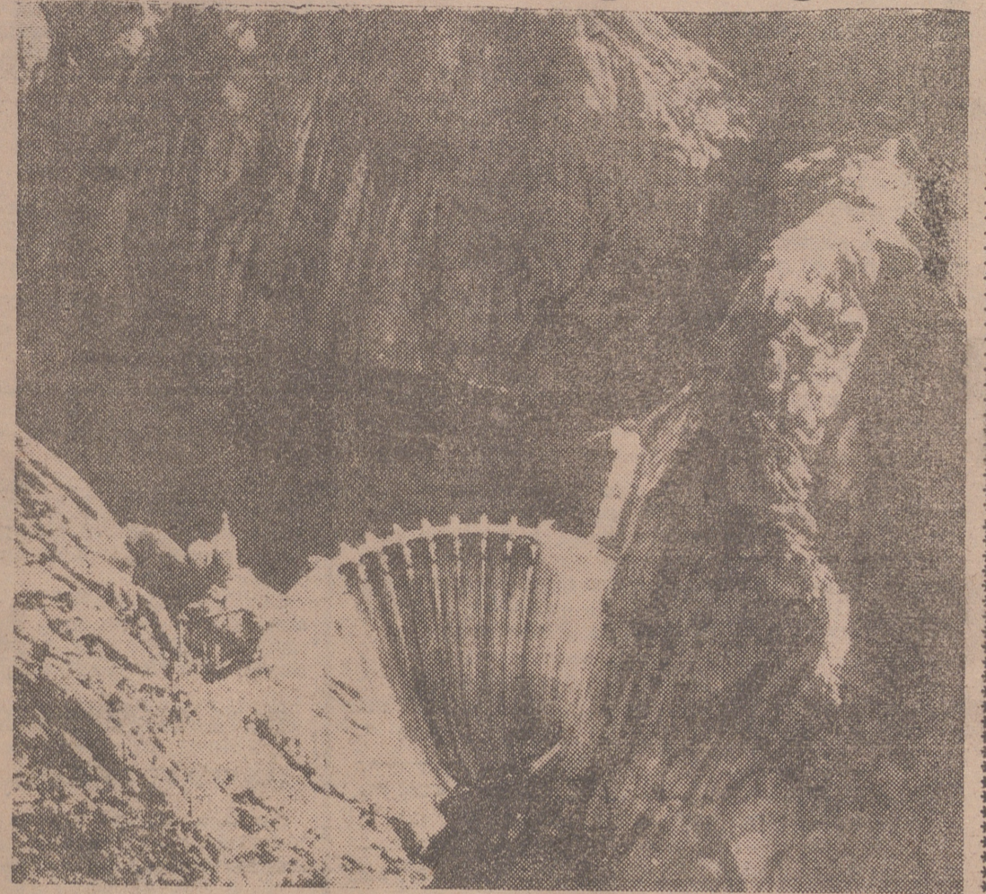
Impresionante vista aérea del Salto de Aldeadávila (Salamanca) que el próximo día 17 será inaugurado por los jefes de Estado de España y Portugal. El Salto, el mayor aprovechamiento hidroeléctrico de Europa Occidental, es una gigantesca empresa con cerca de cuarenta años de historia.—(Foto Fiel).
