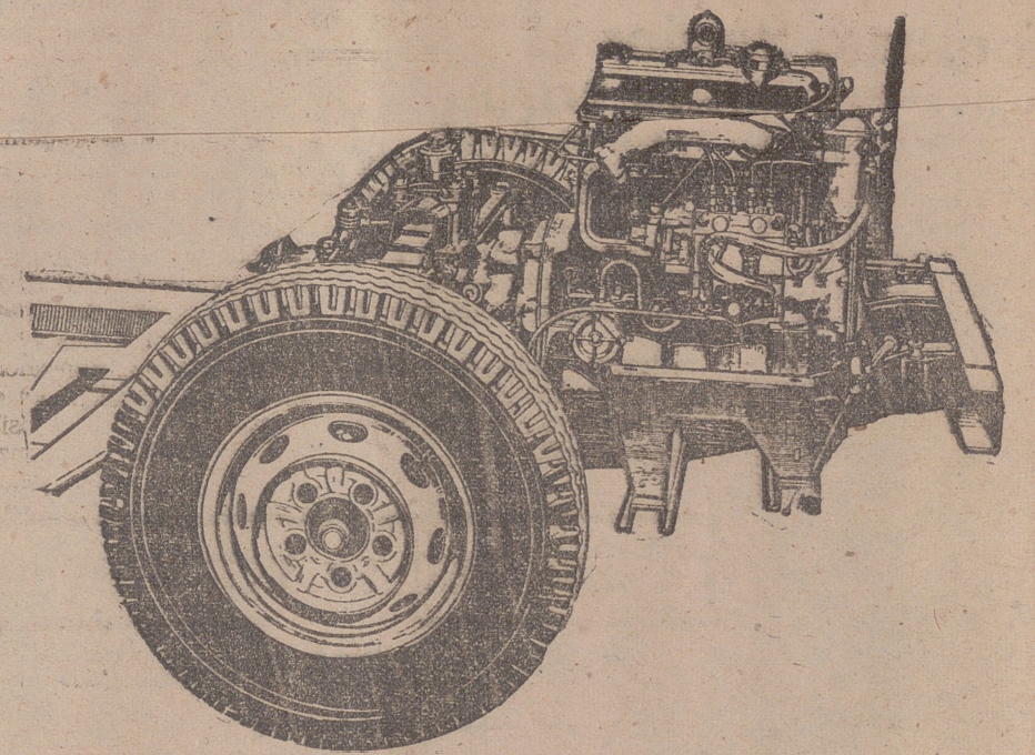
Dibujo que muestra al detalle el motor Mercedes-Benz, con el que va equipada la DKW en su versión Diesel.
