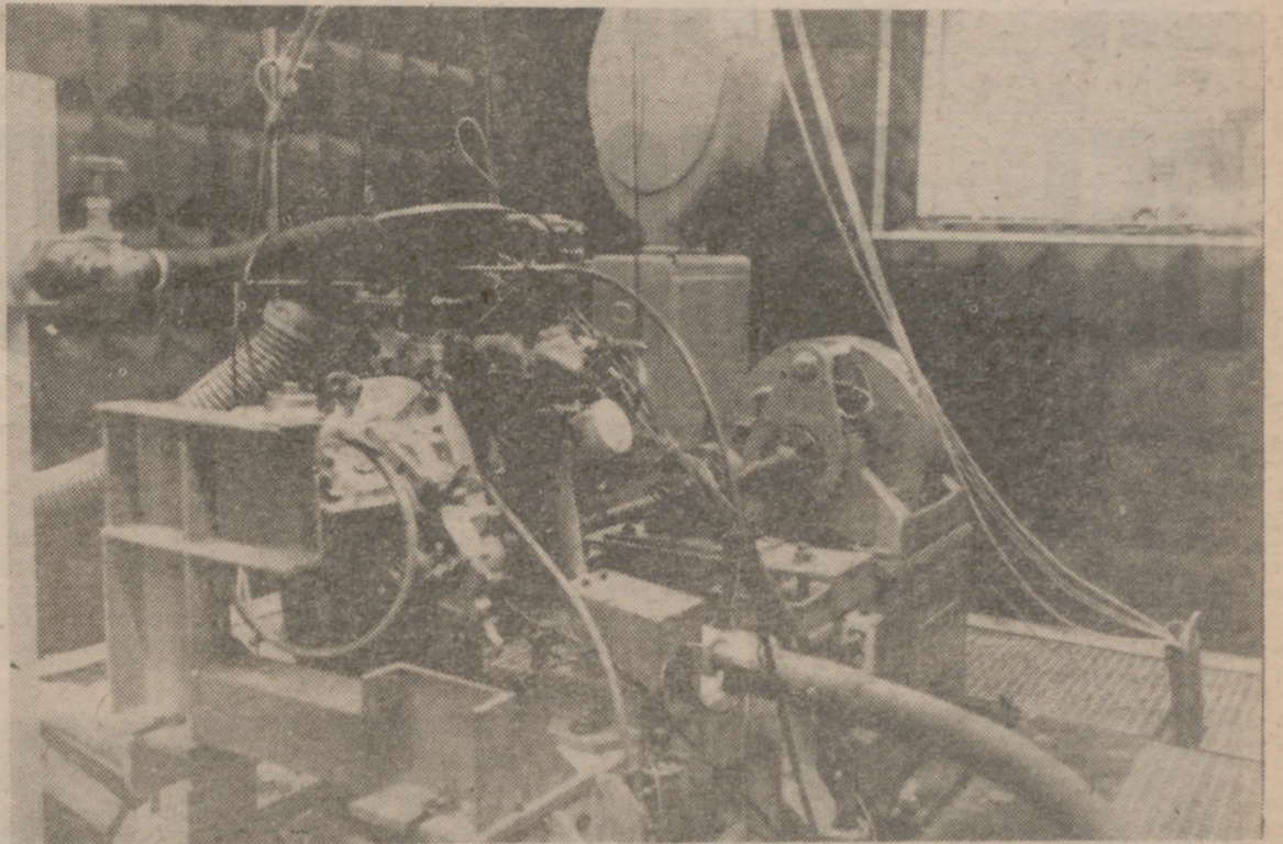
Prueba en banc del motor del "127 Especial", con 1.010 c. c. y 52 CV (DIN), derivado del clásico "903", según proyecto propio del Centro Técnico Seat, en Martorell.—(Foto PYRESA.)
