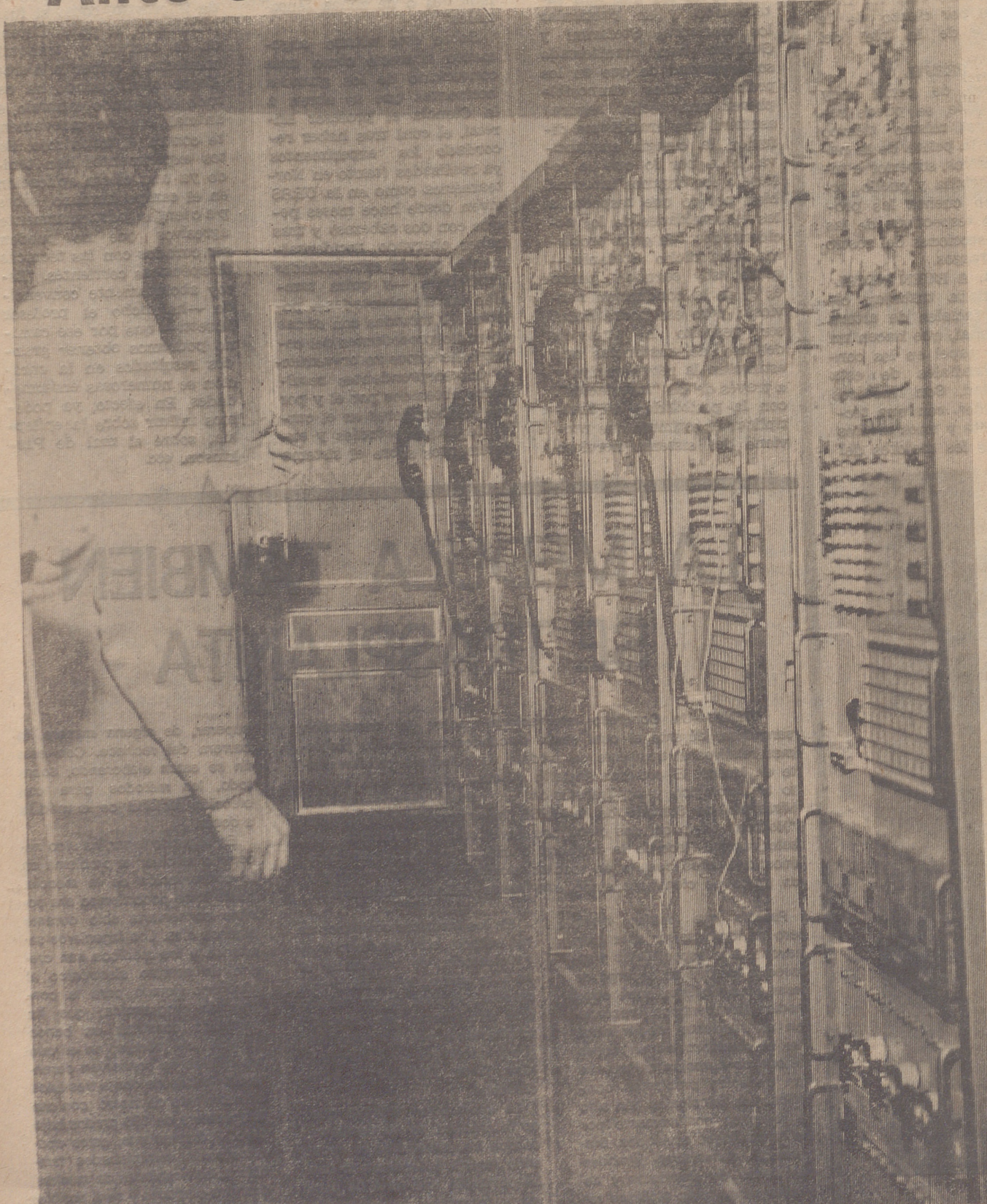
Central automática telefónica con trescientas líneas que ha sido instalada en el Teatro Real con motivo de dicho gran acontecimiento. — (Foto «Cifra-Gráfica»).
