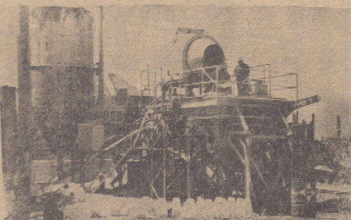
Planta de hormigonado de Santo Domingo.
