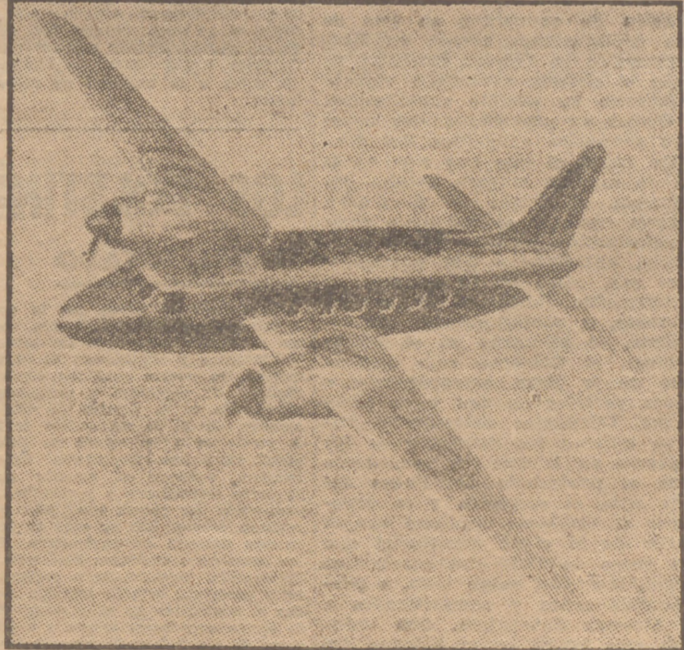
Fotografía del primer avión bimotor Viking VC-1, de la firma inglesa Armstrong-Vickers, llegado hoy al aeródromo de Barajas en su primer vuelo comercial procedente de Londres. Va equipado con dos motores Bristol de 1.675 HP, tipo Hercules 130. Tiene capacidad para treinta pasajeros. (Foto Galpa.)
