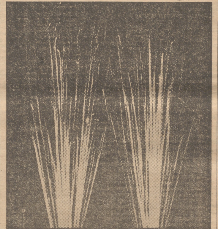
Partículas rápidas procedentes de la desintegración de las que se han servido los científicos para dividir el átomo. Las colisiones se señalan por las desviaciones de los rayos.
