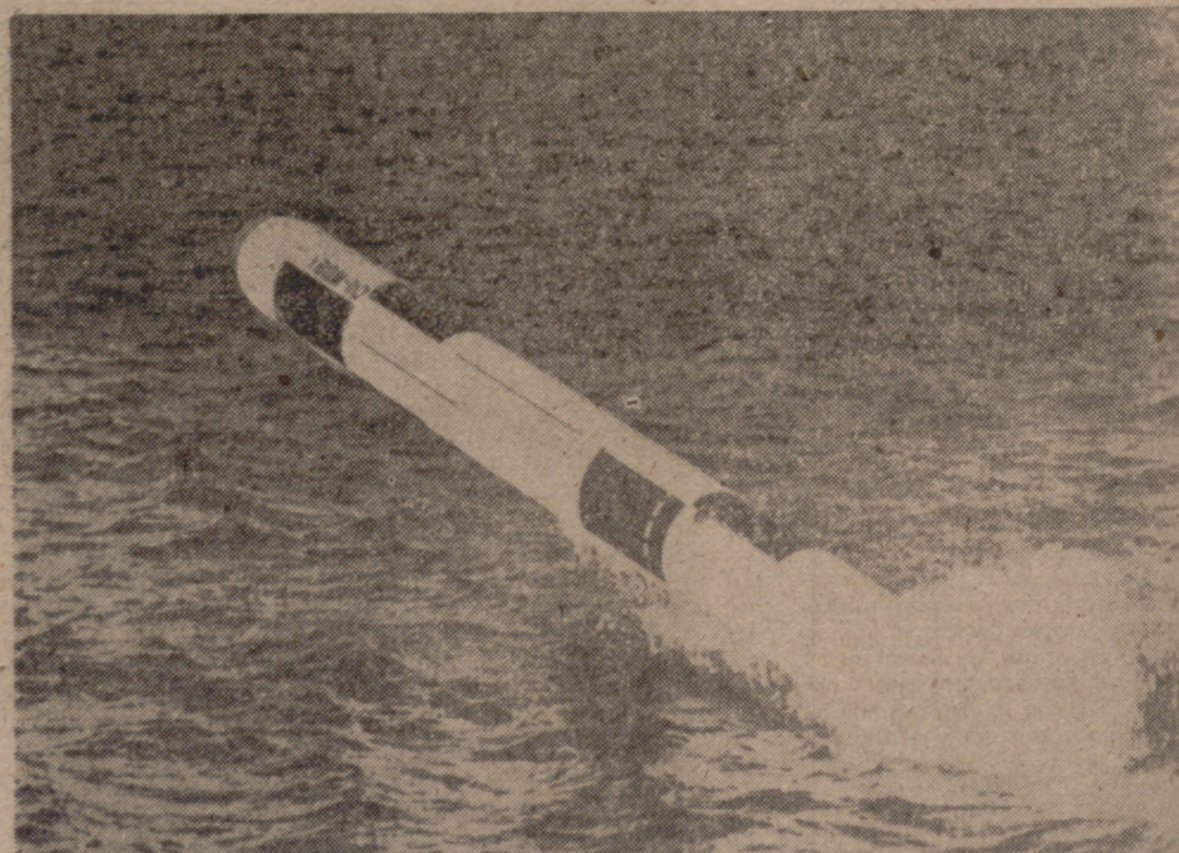
SAN CLEMENTE (California)—Prueba de un nuevo proyectil dirigido para la Marina, diseñado por el laboratorio aerospacial de Dallas. El cohete es disparado bajo el agua, impulsado por un pequeño motor, pero una vez fuera extiende unas alas y es potentemente impulsado para alcanzar largas distancias.—(Telefoto Cifra Gráfica-Upi.)
