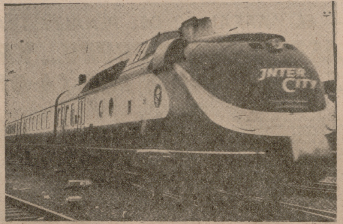
LUDWIGSHAFEN.—(DaD).—Los ferrocarriles federales alemanes acaban de poner en servicio el primer tren de viajeros propulsado por turbinas de gas, el cual enlaza diariamente las ciudades de Ludwigshafen, situada al sur de Frankfurt del Meno y Hamburgo, al norte de la República Federal de Alemania. La locomotora tiene una potencia de 4.400 Cv., lo que le permite realizar una velocidad media de 160 kilómetros por hora. Este nuevo tren de turbina de gas irá reemplazando con el tiempo al tren Diesel en todas las líneas de larga distancia, ya que los 2.200 Cv. de potencia del motor Diesel no son suficientes para mantener una velocidad media que resulte competitiva con la aviación comercial interurbana.
