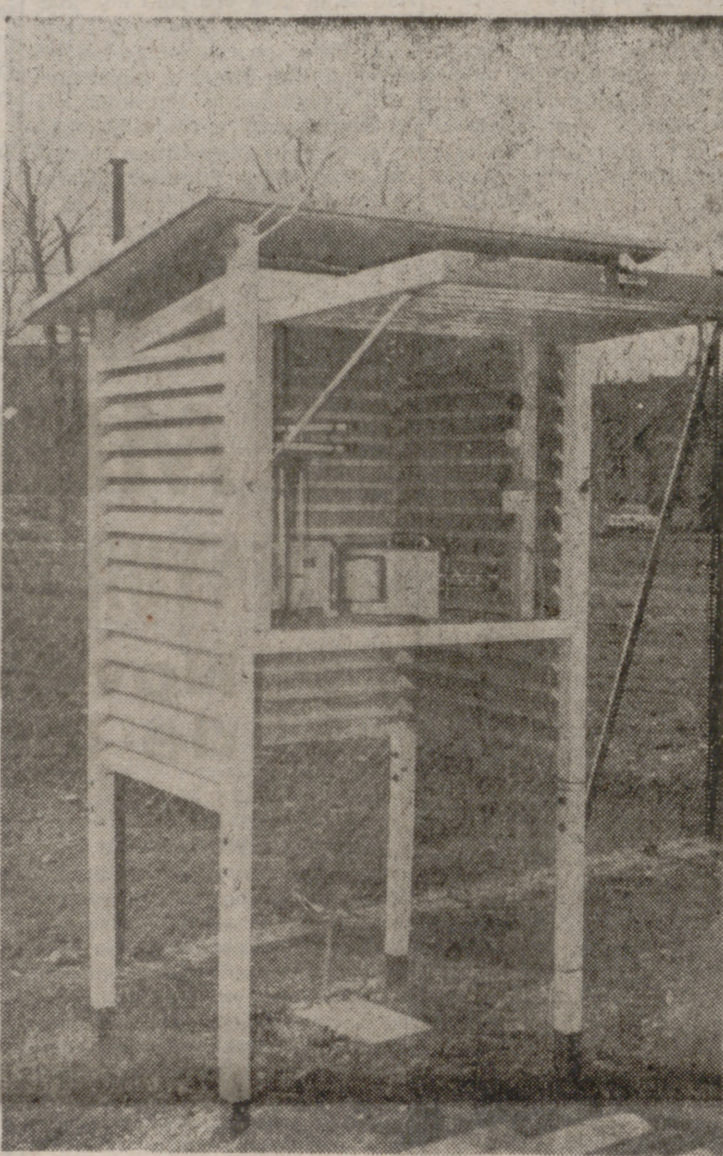
La garita o abrigo meteorológico. En su interior se pueden ver el termógrafo, higrógrafo, termómetro de máxima y mínima, evaporímetro y psicrómetro.
