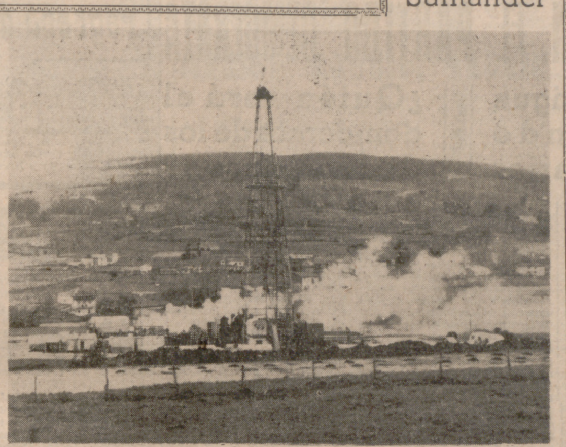
MERUELO. (Santander). — Torre de perforación y otras instalaciones montadas en este pueblo con motivo de los trabajos de sondeo y prospección petrolífera que se llevan a cabo desde hace un mes. — (Foto Cifra Gráfica.)
