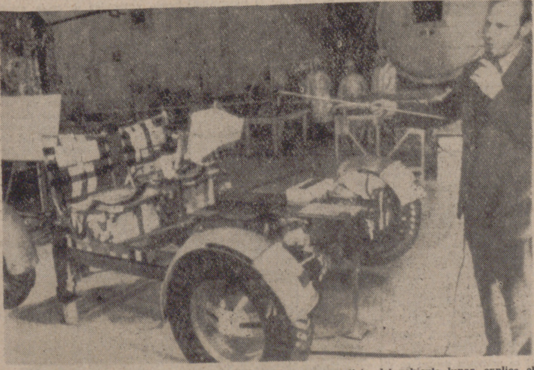
CABO KENNEDY (Florida).— Lindsey Bolton, ingeniero proyectista del vehículo lunar, explica el diseño junto a un modelo del mismo. El vehículo será usado para transportar a los cosmonautas del "Apolo XV" por la Luna, durante su misión prevista para el 26 de julio. — (Telefoto Cifra.)
