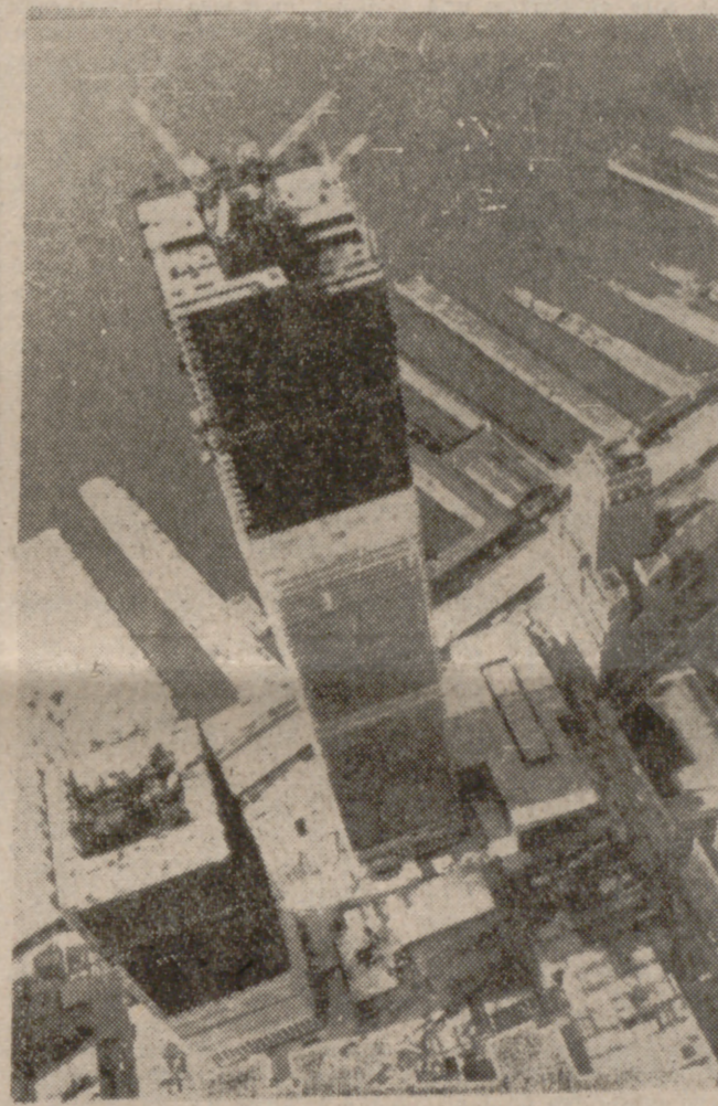
NUEVA YORK. — El edificio del "World Trade Center" ("Centro Comercial Mundial"), actualmente en construcción, es el más alto del mundo, habiendo rebasado al famoso "Empire State". Cuando quede terminado tendrá ciento diez pisos. (Foto Cifra Gráfica.)
