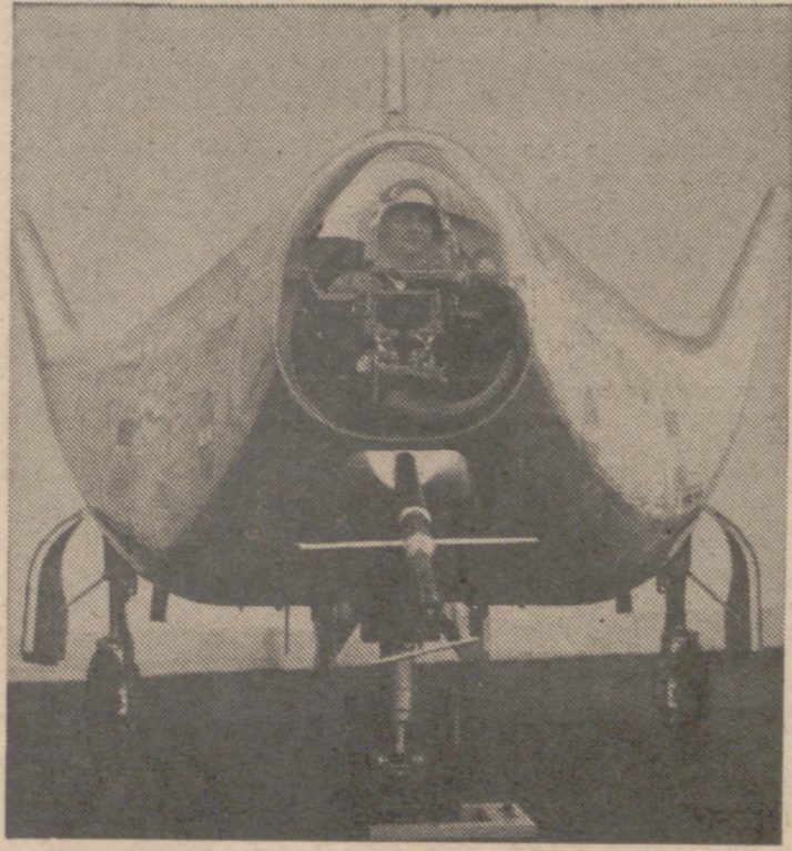
El piloto experimental de los Estados Unidos, Milton Thompson, aparece sentado en la cabina del HL-10. Este aparato experimental, de tres alas, pero desprovisto de alas, ha sido diseñado para contribuir a resolver los problemas de control de los futuros vehículos espaciales tripulados que regresan a la atmósfera terrestre procedentes de vuelos espaciales profundos.
