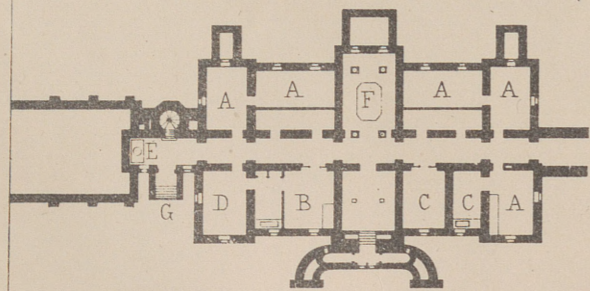
PLAN DV SOVS-SOL.
