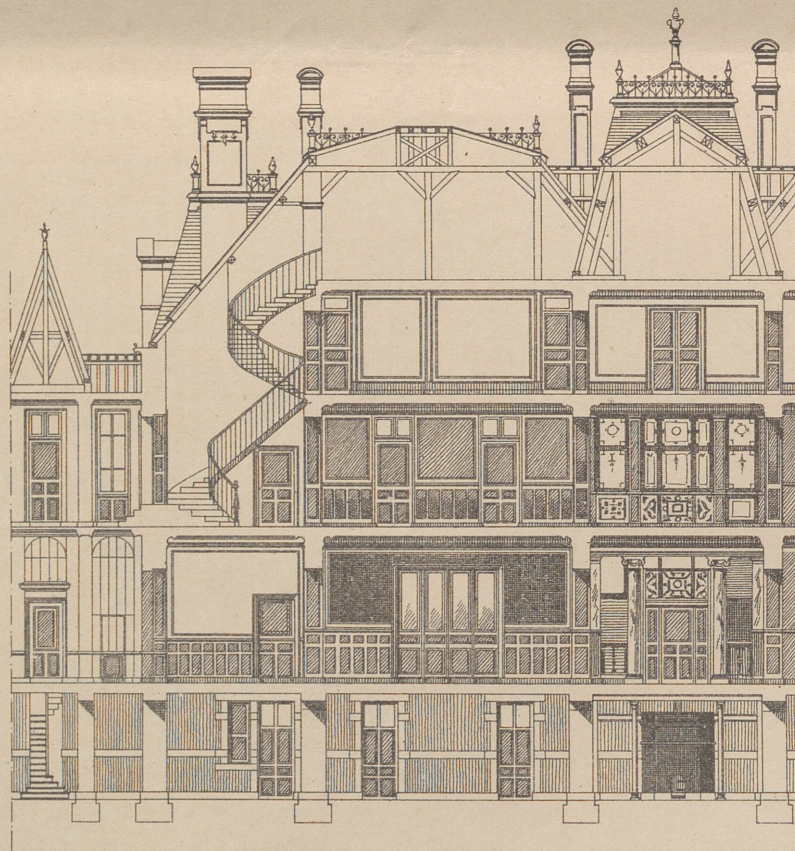
COUPE LONGITUDINALE
