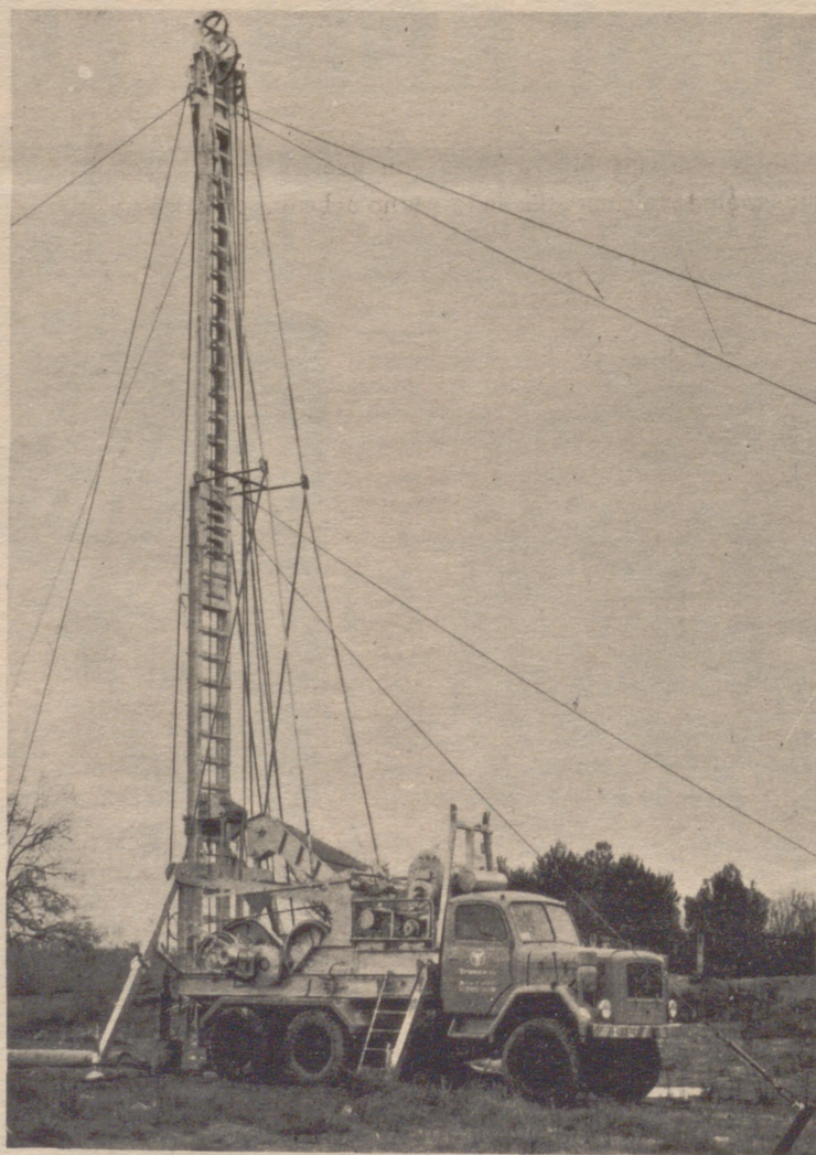
Las perforadoras a percusión por cable son las más normales para la captación del agua subterránea. Pueden alcanzar profundidades de 700 metros o más con diámetro máximo de unos 500 milímetros.
