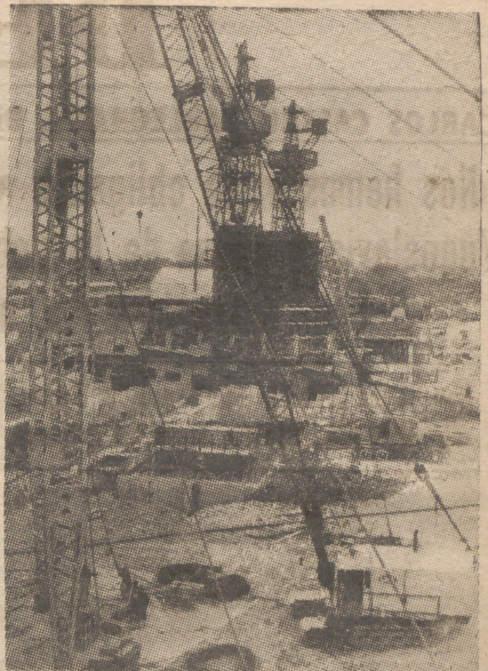
Vista de las obras de la central nuclear de Berkeley. (Foto Europa.)
