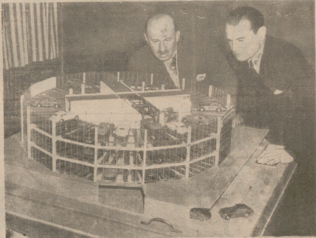
El "Rotapark" es un nuevo modelo de garaje y cuya maqueta se puede apreciar en la fotografía. Fue ideado por los norteamericanos, pero será construido por los ingleses cerca de Southwark Bridge. Los coches entran hasta unos grandes ascensores, en torno a los cuales el garaje va dando vueltas hasta presentar un sitio libre enfrente a la puerta del ascensor accionado. Para retirar el vehículo, lo único que tiene que hacer el conductor es introducir una tarjeta en una máquina electrónica, y el proceso se repite a la inversa. Con esta modernísima jaula para coches, cuyo funcionamiento ha de constituir un espectáculo atractivo, se han terminado los problemas de aparcamiento. La verdad es que, con tan cómodas soluciones, el mundo va a quedar aburridísimo... (Foto Keystone-Nemes.)
