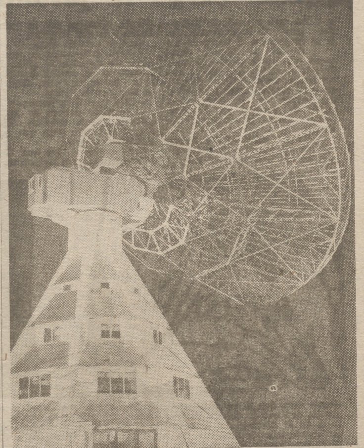
En la Alemania occidental, y no muy lejos de Bonn, funciona ya este gigantesco radiotelescopio, instalado en lo alto de la montaña Stockert. Percibe las radiaciones de millones de estrellas, en especial las de la Vía Láctea, con lo que se amplía considerablemente el campo de las investigaciones astronómicas. El gran reflector parabólico, que aparece en la fotografía, es un gigantesco aparato de radio que capta las emisiones de ondas que lanzan los astros. (Foto Keystone-Nemes.)
