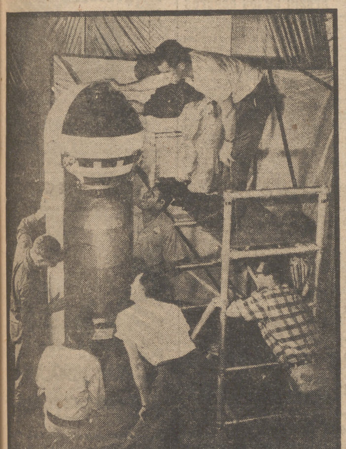
EL «PIONEER V» SE PREPARO ASI Continúa su recorrido en la órbita solar el planeoide artificial norteamericano «Pioneer V», que actualmente lleva una velocidad superior a los 8.000 kilómetros por hora, y que la irá aumentando progresivamente bajo la influencia de la gravedad del sistema solar, para alcanzar la máxima hacia el 10 de agosto, fecha en que se hallará más cerca del astro. En la fotografía, técnicos norteamericanos de la base de Cabo Cañaveral (Florida) realizan los últimos preparativos en la tercera parte del cohete del «Pioneer V», momentos antes de que estuviera dispuesto para su lanzamiento.
