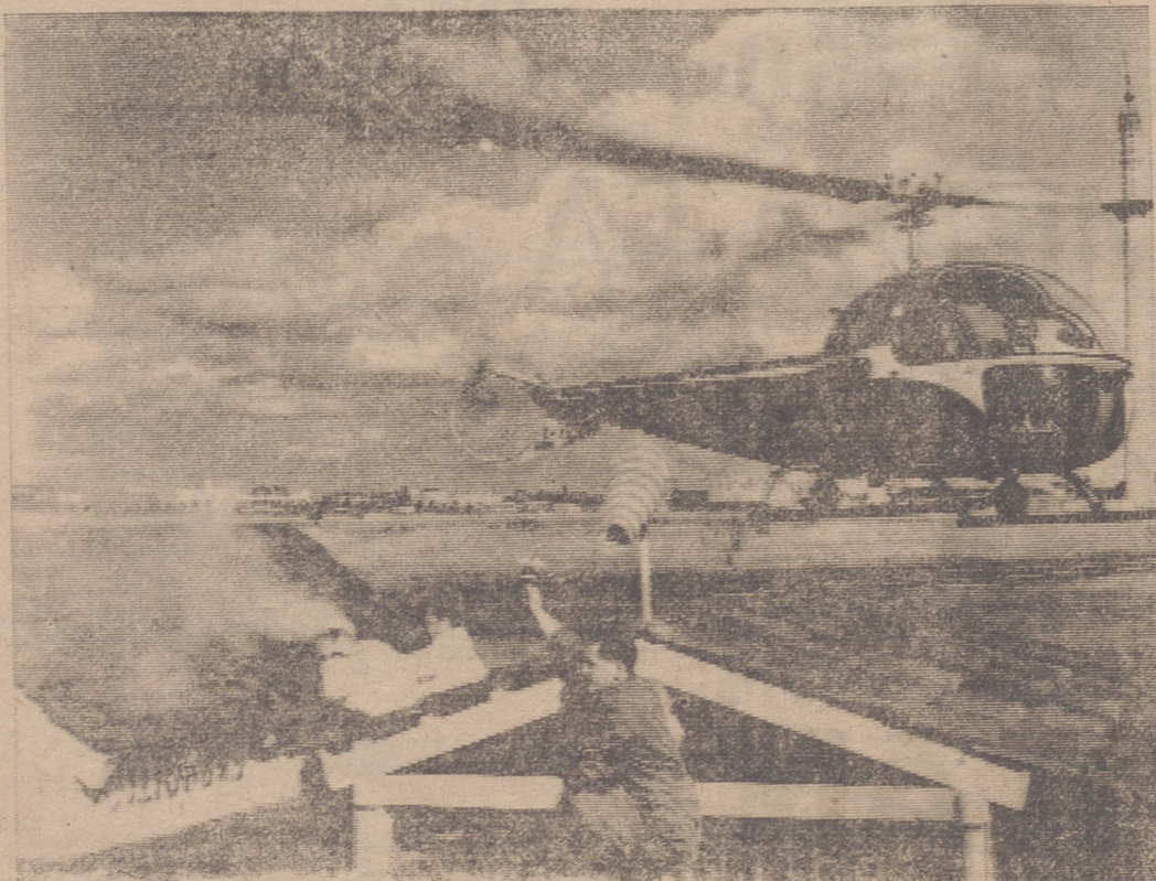
Para medir la resistencia contra el viento se han realizado varias pruebas con ayuda de un helicóptero de los tejados que habrán de instalarse en la Ciudad Olímpica de Munich. El resultado ha sido favorable. Las tejas no volarán. (Foto "Fiel")
