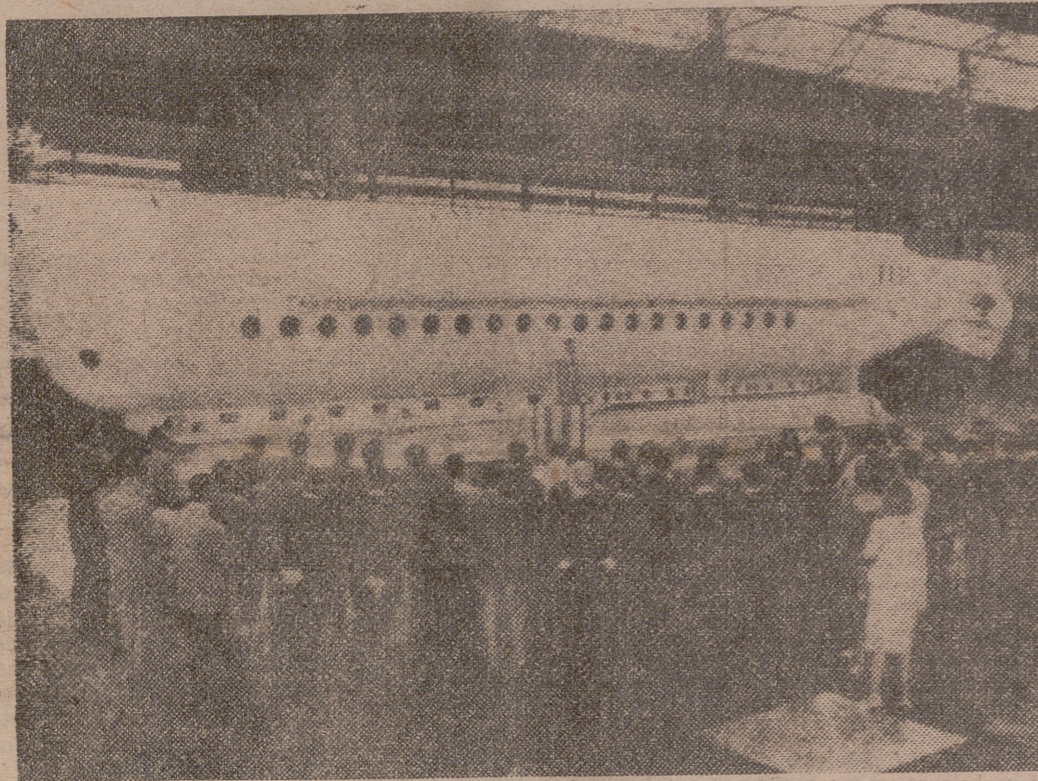
La construcción exterior del "Mesoscafo", el primer submarino turístico, ha terminado, y Jacques Piccard, su constructor, presenta el submarino a la Prensa y explica los datos técnicos del mismo. —(Foto "Fiel").
