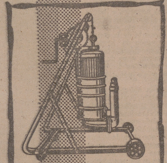
BOMBA LETRIN para elevación y trasego de líquidos densos, mostos, pulpas, etc.
