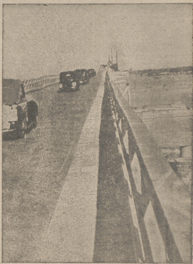
El mayor puente de guerra construido por la Organización Todt en el frente del Este ha sido abierto al tráfico. A pesar de los grandes frios y hielos se trabajó día y noche en él para lograr en el plazo previsto su terminación. Este puente tiene una longitud de unos mil quinientos metros
