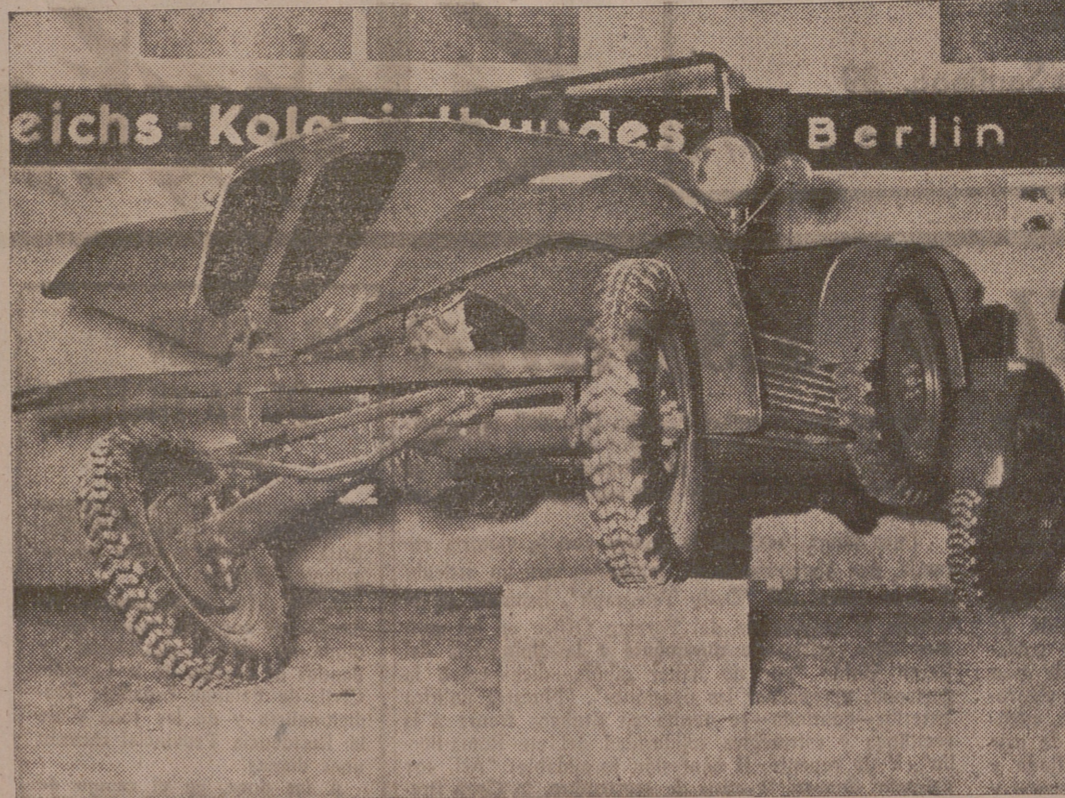
Un automóvil ideal para toda clase de terrenos, apropiado para regiones de la zona tropical y de ultramar. La adaptación a terreno accidentado es sorprendente, y esto a causa de la construcción especial del coche
