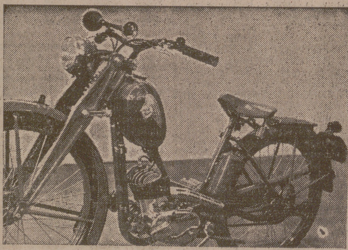
Una motocicleta del tipo ligero, para señoras, construida por la conocida fábrica «Ligtel y Sachs».
