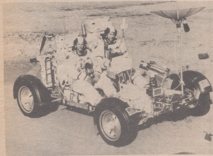
Los astronautas John W. Young (derecha) y Charles M. Duke, Jr., maniobran con una versión de pruebas del vehículo diseñado para andar por la Luna, llamado "rover", haciéndolo por un terreno que tiene características parecidas a las de la superficie de la Luna. La antena en forma de plato será utilizada para transmitir a la Tierra imágenes de televisión en color mientras el vehículo esté aparcado en la Luna. La cámara de televisión, que va en el centro de la parte delantera del vehículo puede ser controlada por radiomando desde el Control de la Misión en Houston (Texas), de forma que las imágenes puedan ser recibidas en la Tierra mientras los astronautas están realizando su trabajo de investigación a alguna distancia del "rover". Este, con su cámara de televisión vuelta, quedará en la Luna de forma que los telespectadores puedan ver el despegue del módulo lunar y la terminación de la excursión por el planeta.
