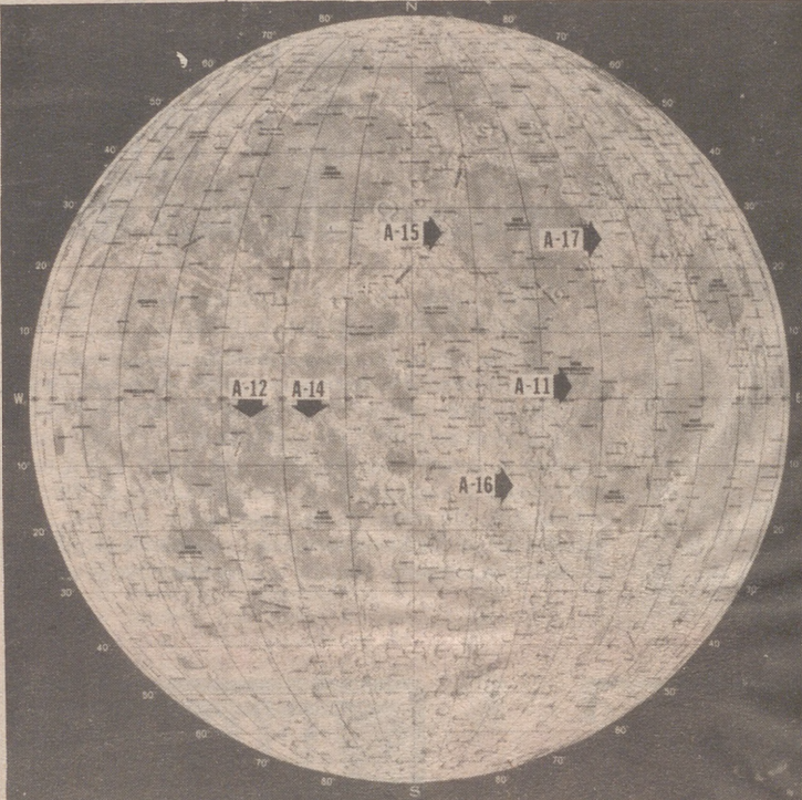
Lugares de aterrizaje de los Apolos.— Este mapa de la Luna muestra los lugares de aterrizaje de los Apolos. Se calcula que la tripulación del Apolo-16 explorará las tierras altas de Descartes en abril de 1972 y el objetivo para el vuelo del Apolo-17 en diciembre de 1972 es el Mar de la Serenidad. Los anteriores vuelos realizados son: el Apolo-11 en el Mar de la Tranquilidad, en julio de 1969; el Apolo-12 en el Océano de las Tormentas, en noviembre de 1969; el Apolo-14 en las tierras altas de Fra Mauro, en febrero de 1971 y el Apolo-15 en la región de los Montes Apeninos-Garganta Hadley, en agosto de 1971. Los astronautas del Apolo-13 circundaron la Luna y regresaron sin aterrizar en su superficie a causa de un mal funcionamiento de su nave espacial.
