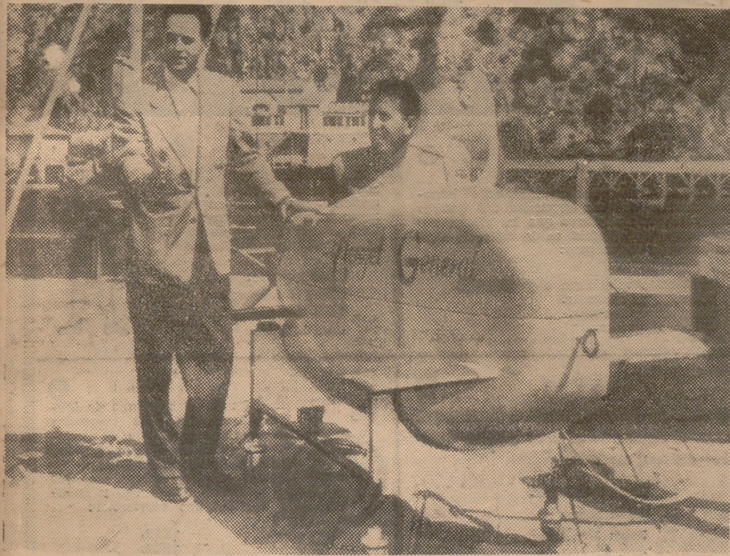
El coinventor del "Minisub", C. A. Congwer, dando instrucciones al "piloto de pruebas", Harold F. Osborne, técnico en natación submarina, para tripular el aparato. (Foto Cifra.)
